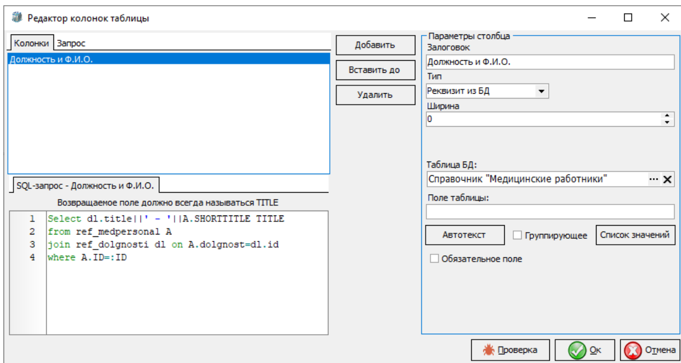
Рисунок 2 – SQL-запрос у типа «Реквизит из БД»
